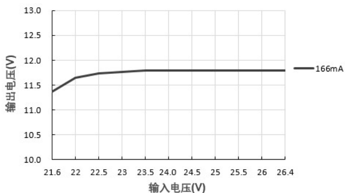
输出电压Vs输入电压 (PS02-B24SS12)
