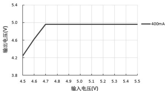
输出电压Vs输入电压 (PS02-B12SS05)
