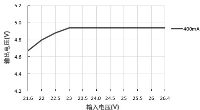
输出电压Vs输入电压 (PS02-B24SS05)
